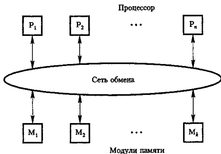
Рис. 12.2. Мультимикропроцессорная система типа UMA
