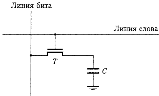
Рис. 5.6. Однотранзисторная ячейка динамической памяти
