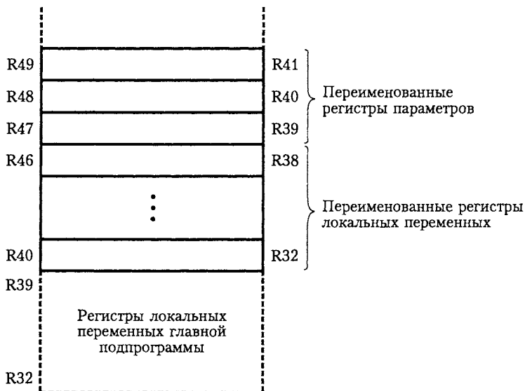
Рис. 11.4. Выделение пространства в стеке регистров для локальных переменных и передачи параметров в архитектуре IA-64: активная область стека регистров в главной программе после выполнения команды Алloc 8,4 (а); активная область стека регистров в подпрограмме после выполнения команды Алloc 7,3 (б)
