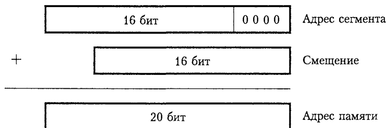
Рис. 11.1. Формирование адреса памяти в процессоре 8086
