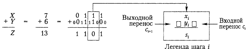
Рис. 6.1. Логическая спецификация одного шага двоичного сложения
