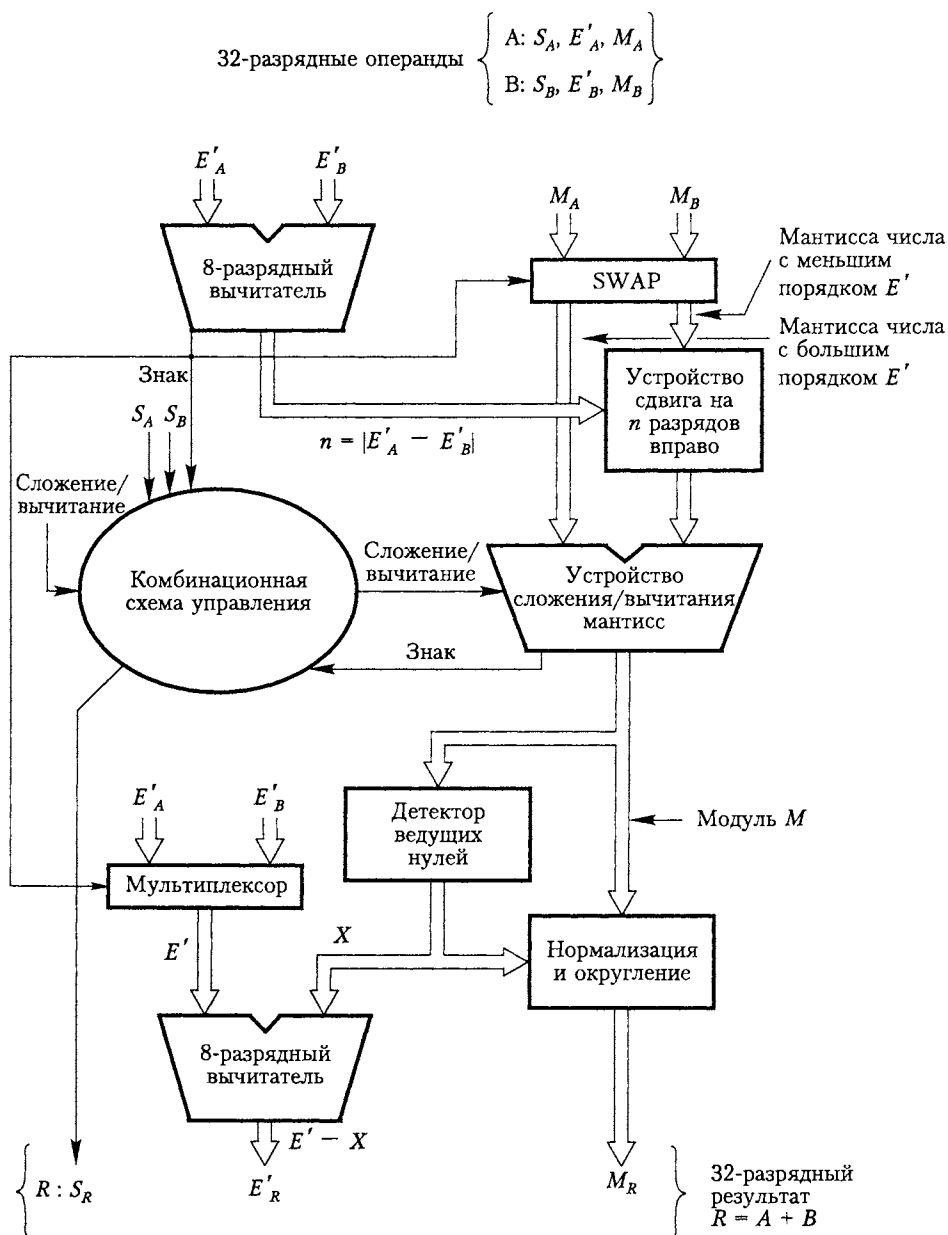
Рис. 6.26. Устройство сложения/вычитания чисел с плавающей запятой
