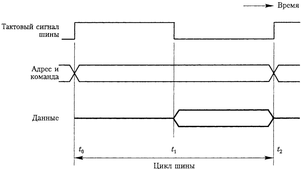
Рис. 4.23. Временная диаграмма операции пересылки по синхронной шине при вводе данных
