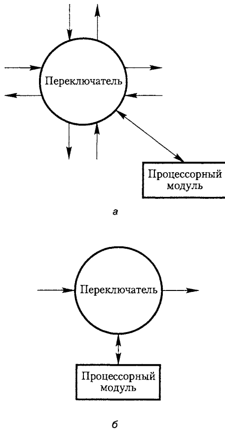
Рис. 12.11. Узлы в различных сетях: узел ячеистой сети (а); узел кольцевой сети (б)
