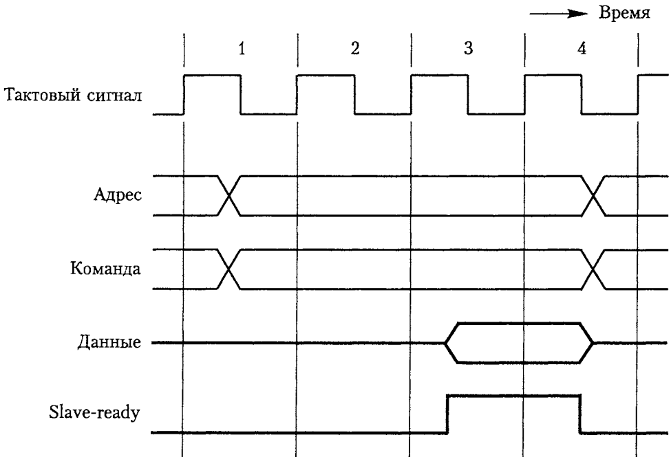
Рис. 4.25. Пересылка данных с использованием нескольких тактов
