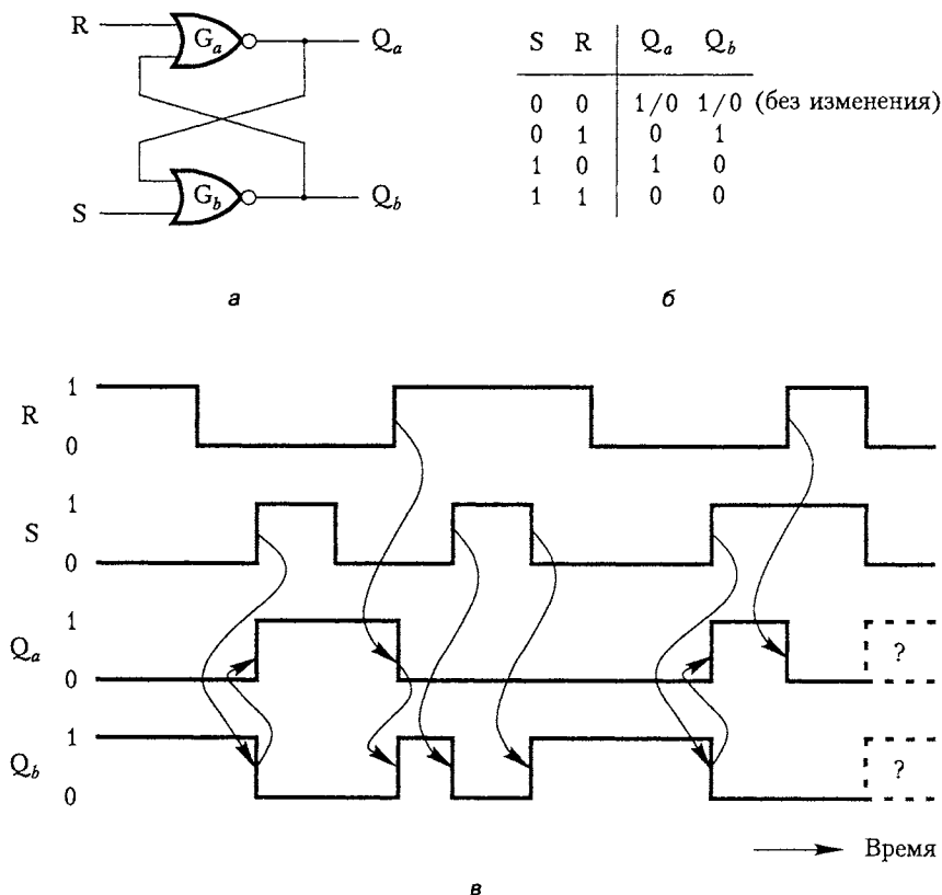
Рис. А.24. Защелка на основе вентилей ИЛИ-НЕ: логическая схема (а); таблица истинности (б); временная диаграмма (в)
