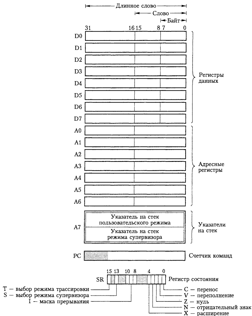
Рис. 3.18. Регистры процессора 68000
