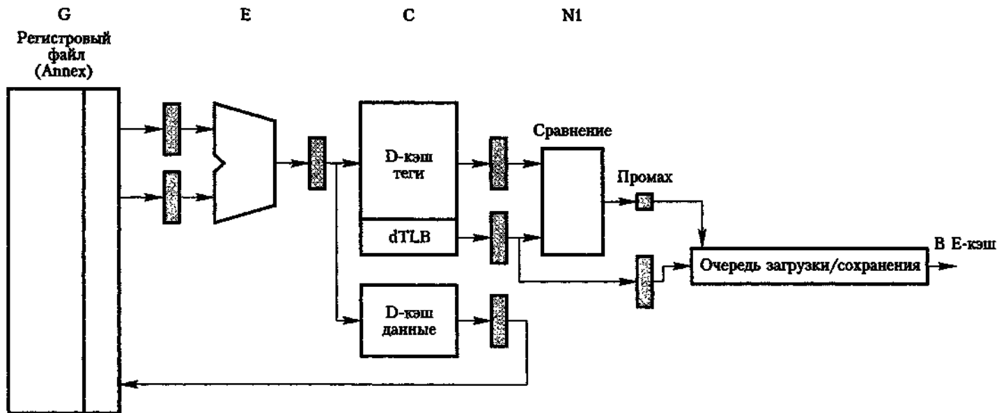
Рис. 8.29. Блок загрузки/сохранения
