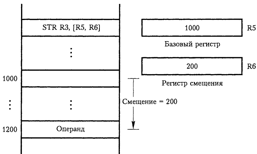
Рис. 3.3. Примеры режимов адресации процессора ARM: относительный (а), преиндексный (б)
