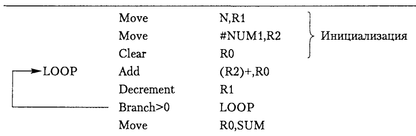
Рис. 2.16. Автоинкрементная адресация в программе, представленной на рис. 2.12
