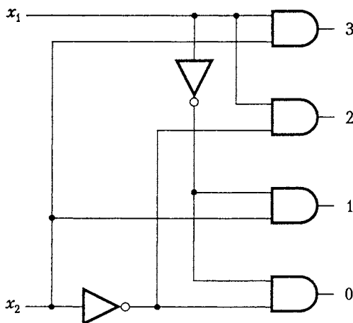
Рис. А.36. Дешифратор с двумя входами и четырьмя выходами
