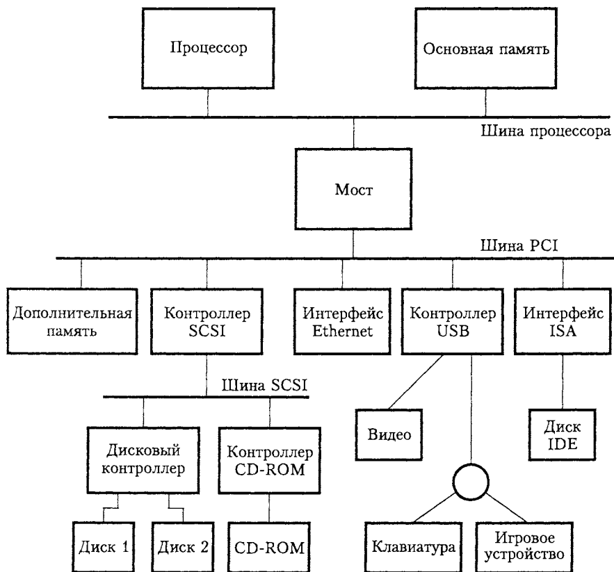
Рис. 4.38. Пример компьютерной системы, в которой используется несколько стандартов интерфейса
