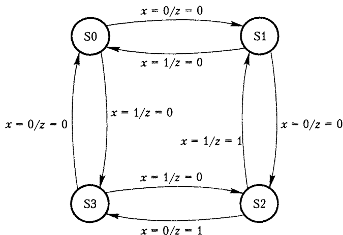
Рис. А.47. Диаграмма состояния для счетчика с прямым/обратным счетом по модулю 4, сигнализирующего о значении 2
