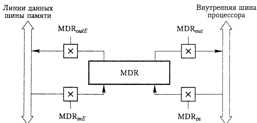
Рис. 7.4. Соединения и управляющие сигналы регистра MDR
