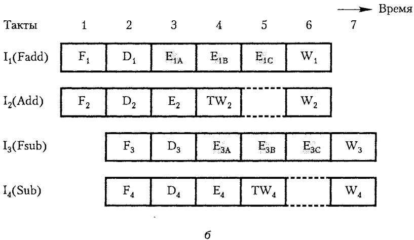
Рис. 8.21. Завершение работы команд в соответствии с порядком их следования в программе: отложенная запись (а); использование временных регистров (б)
