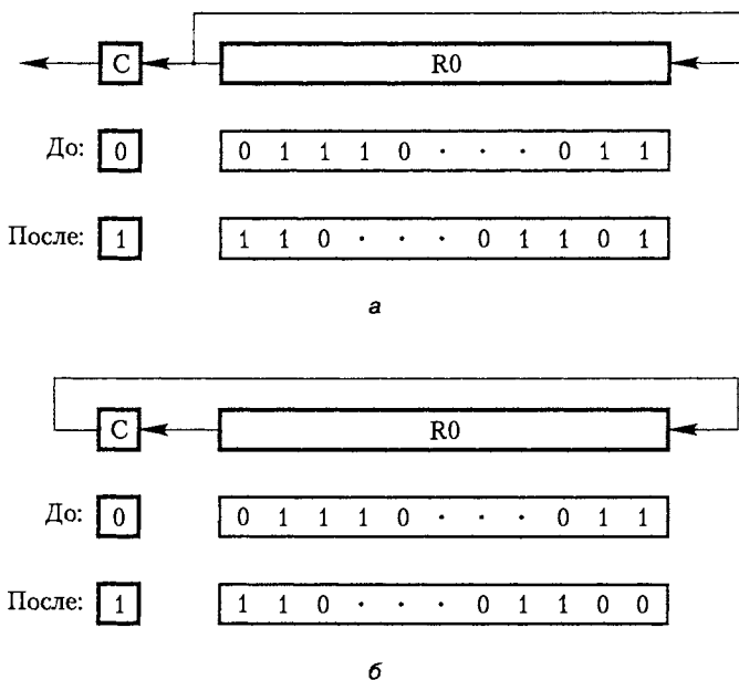
Рис. 2.32. Команды циклического сдвига: влево без переноса, RotateL #2,R0 ( а ); влево с переносом, RotateLC #2,R0 ( б ); вправо без переноса, RotateR #2,R0 ( в ); вправо с переносом, RotateRC #2,R0 ( г )
