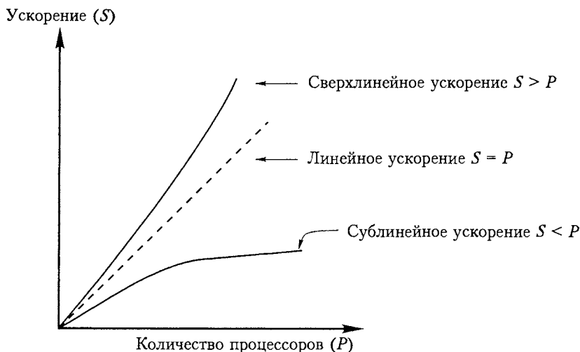
Рис. 12.21. Диаграмма изменения ускорения в мультипроцессорных системах
