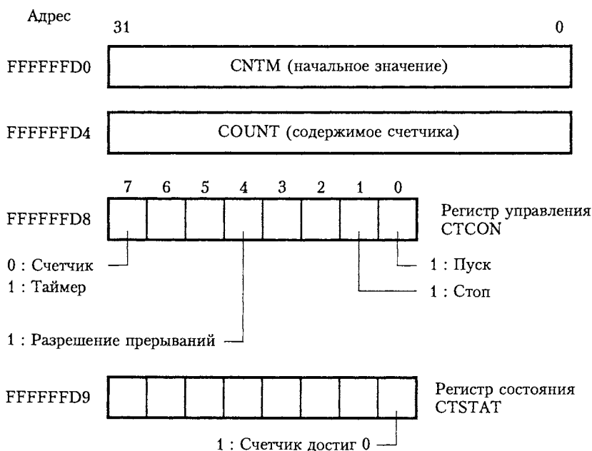
Рис. 9.9. Регистры счетчика/таймера
