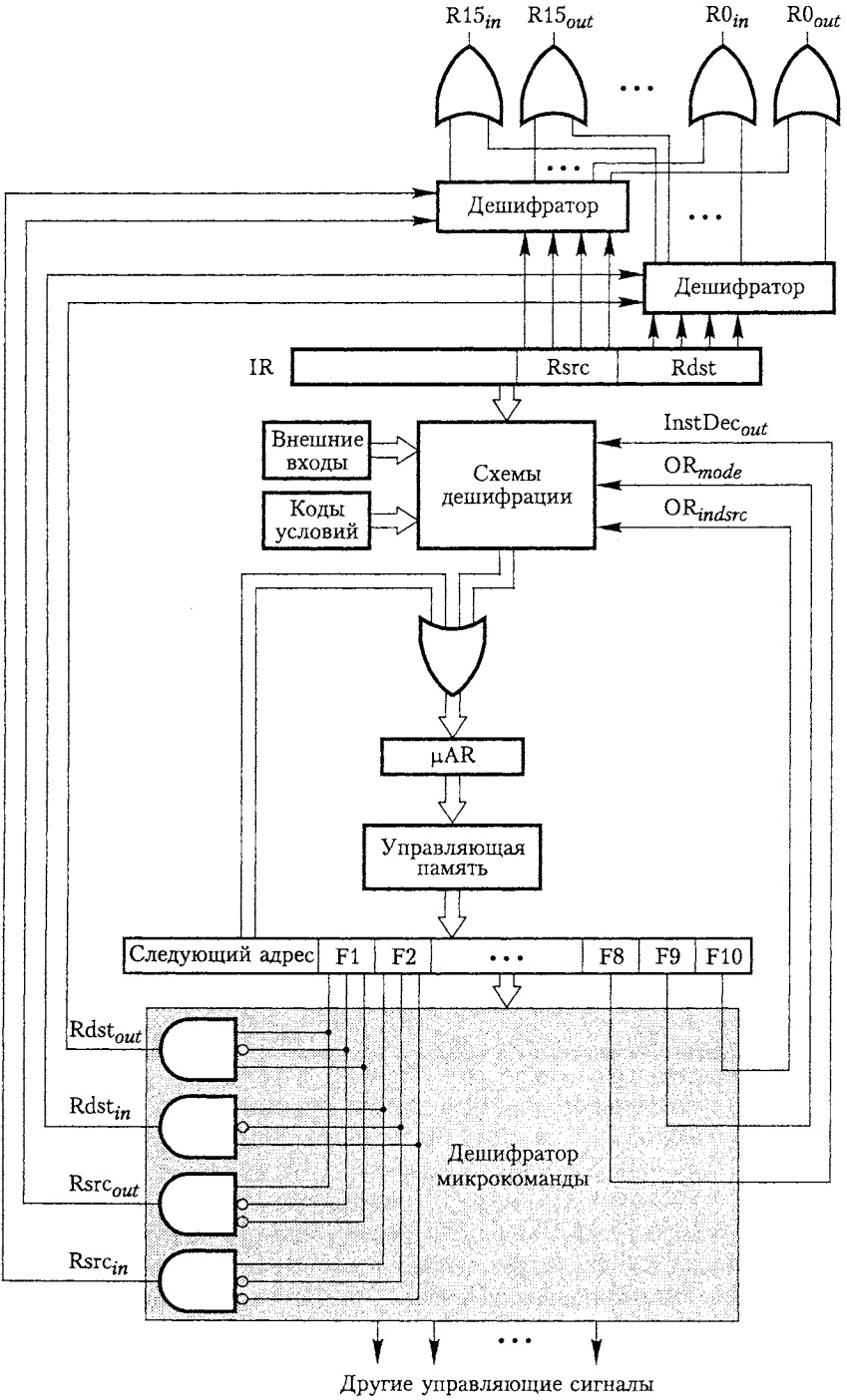
Рис. 7.25. Подробная схема формирования управляющих сигналов
