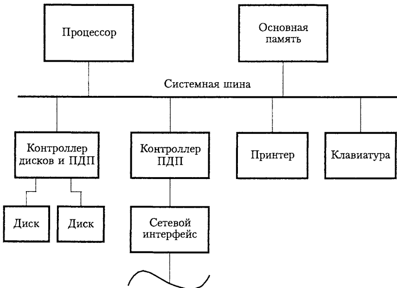
Рис. 4.19. Использование контролеров ПДП в компьютерной системе
