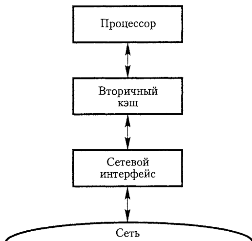
Рис. 12.12. Процессорный узел в мультимикропроцессорной системе, показанной на рис. 12.2
