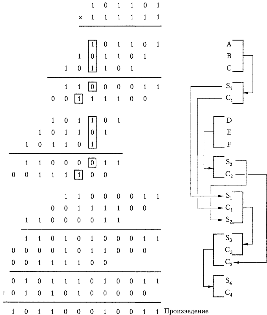
Рис. 6.18. Пример выполнения умножения с использованием операции сложения с сохранением переноса (для примера на рис. 6.17)
