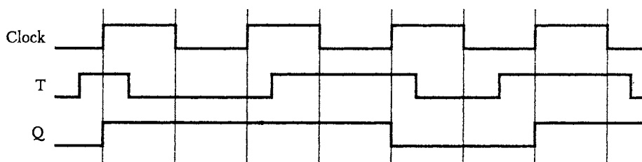
Рис. А.30. Т-триггер: схема (а); таблица истинности (б); графическое обозначение (в); временная диаграмма (г)
