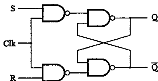
Рис. А.26. Вентильная SR-защелка, реализованная на основе вентилях И-НЕ
