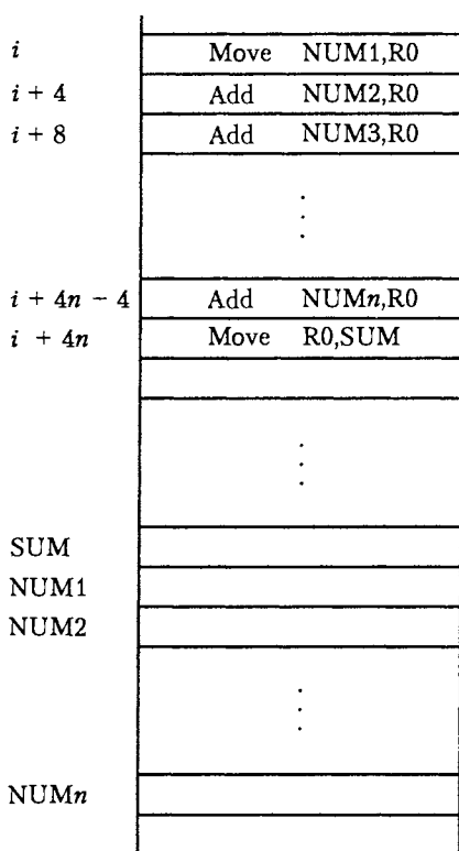
Рис. 2.9. Прямолинейная программа для сложения n чисел
