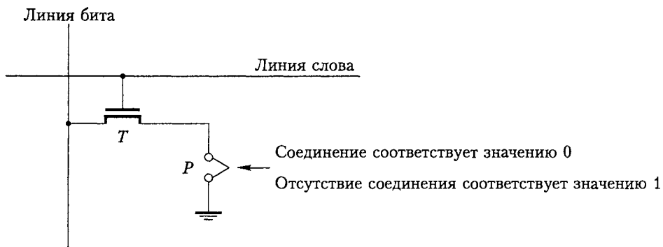
Рис. 5.12. Ячейка PROM
