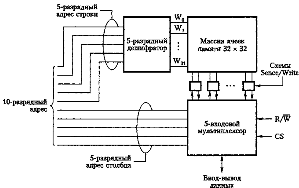
Рис. 5.3. Микросхема памяти 1\text{ К} \times 1
