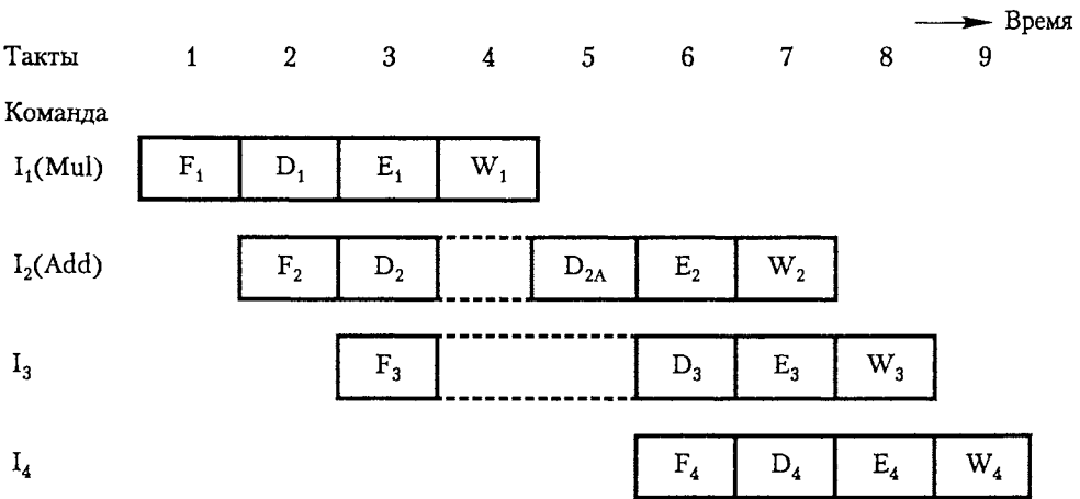
Рис. 8.6. Конвейер приостановлен из-за того, что данные шага D 2 зависят от данных шага W 1
