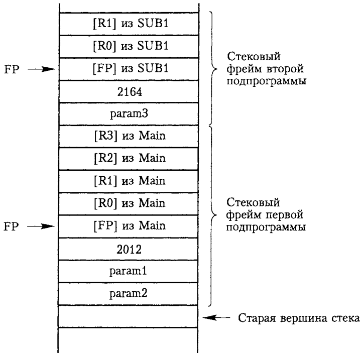
Рис. 2.29. Стековые фреймы программы, приведенной на рис. 2.28
