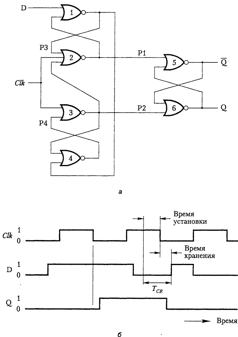
Рис. А.29. D-триггер, тактируемый отрицательным фронтом сигнала: схема (а); пример временной диаграммы (б)
