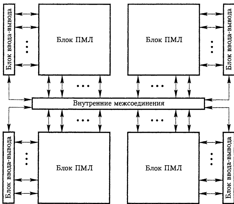
Рис. А.45. Структура сложного программируемого логического устройства
