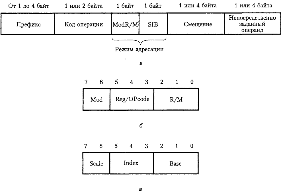
Рис. Г.1. Формат команд IA-32: общий формат (а); байт ModR/M (б); байт SIB (в)
