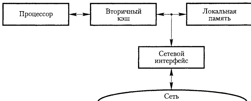
Рис. 12.13. Структура узла мультимикропроцессора, изображенного на рис. 12.3
