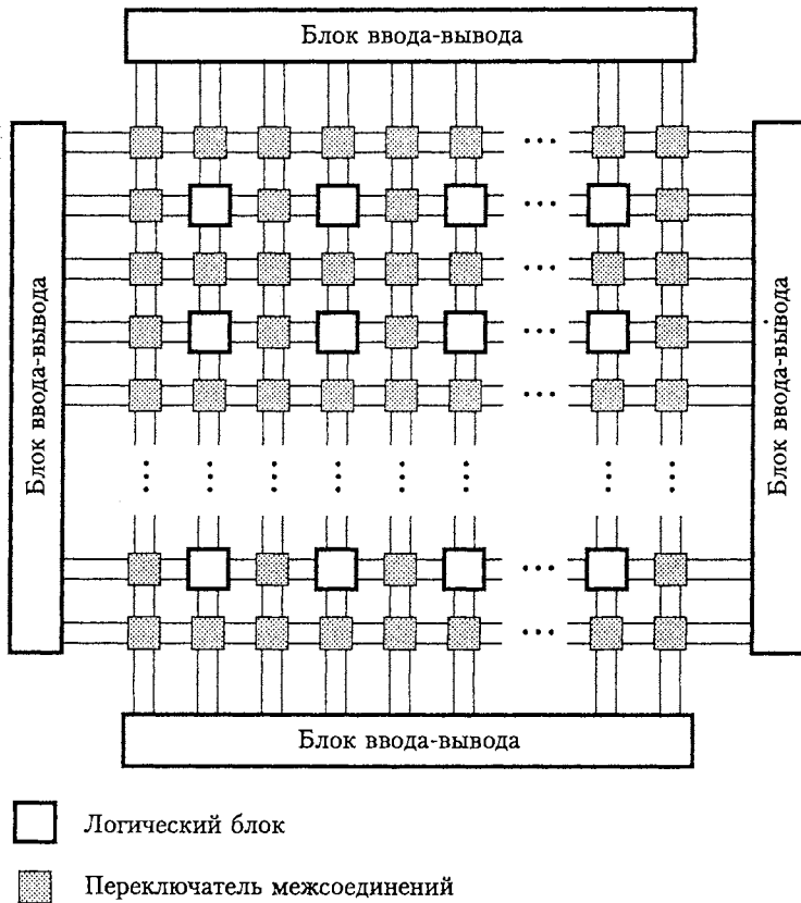
Рис. А.46. Концептуальная схема программируемой вентиляной матрицы
