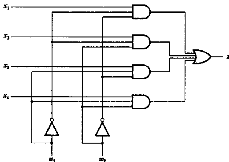
Рис. А.38. Четырехвходовый мультиплексор
