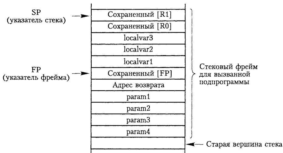
Рис. 2.27. Пример стекового фрейма
