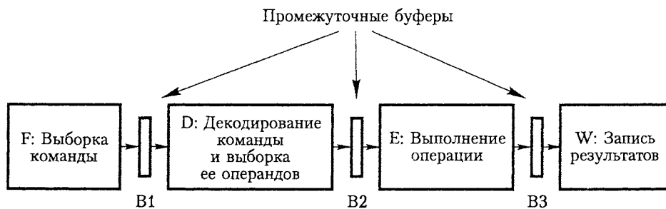
Рис. 8.2. Структура 4-ступенчатого конвейера: выполнение команды за 4 шага (а); аппаратная организация (б)
