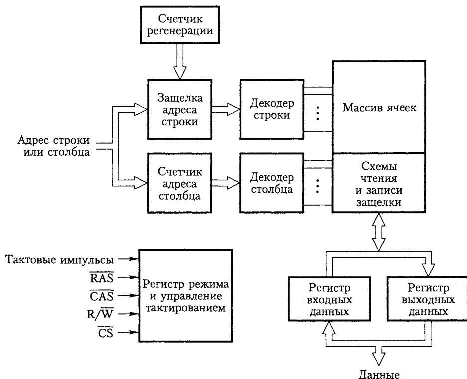
Рис. 5.8. Синхронная DRAM
