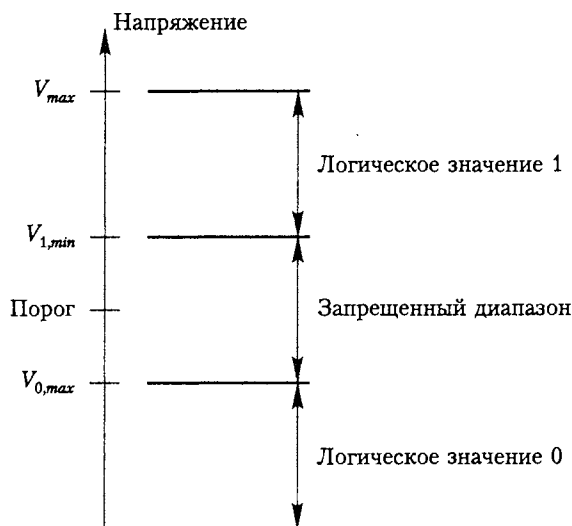
Рис. А.10. Представление логических значений посредством уровней напряжения
