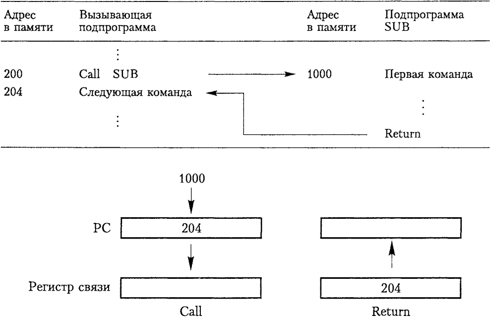
Рис. 2.24. Связывание подпрограммы через регистр связи
