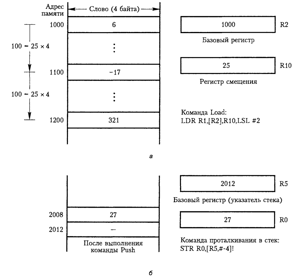
Рис. 3.4. Режимы адресации процессора ARM, в которых используется обратная запись: постиндексный (а); преиндексный (б)
