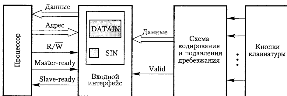
Рис. 4.28. Схема соединения клавиатуры с процессором
