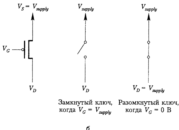
Рис. А.14. Логические схемы транзисторов: n-МОП (а); p-МОП (б)
